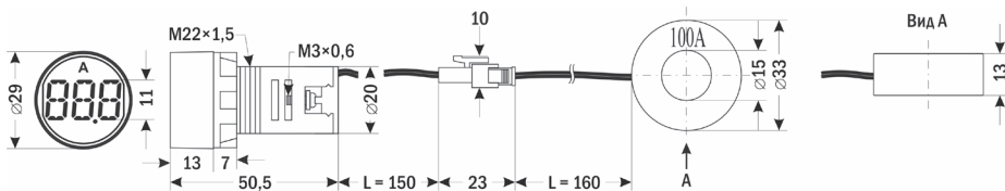
Рис. 6 – Размеры Omix R30-A1-1
