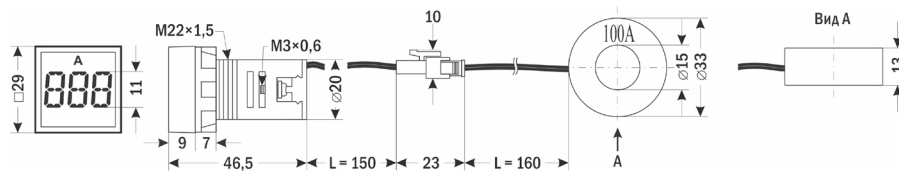
Рис. 7 – Размеры Omix T33-A1-1
